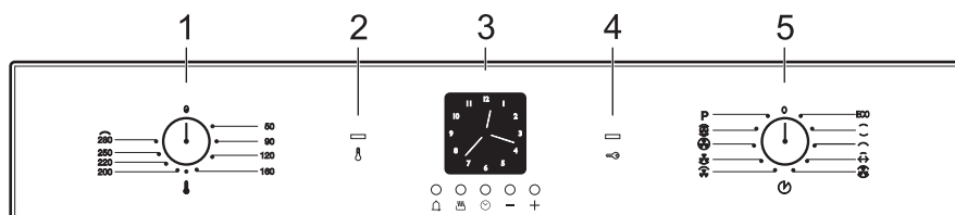
Пиrolитические модели
