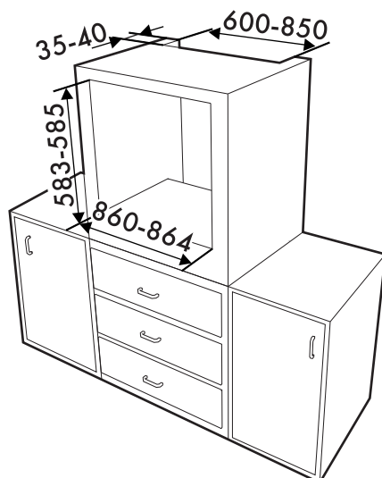
Вертикальное встраивание (мм)
